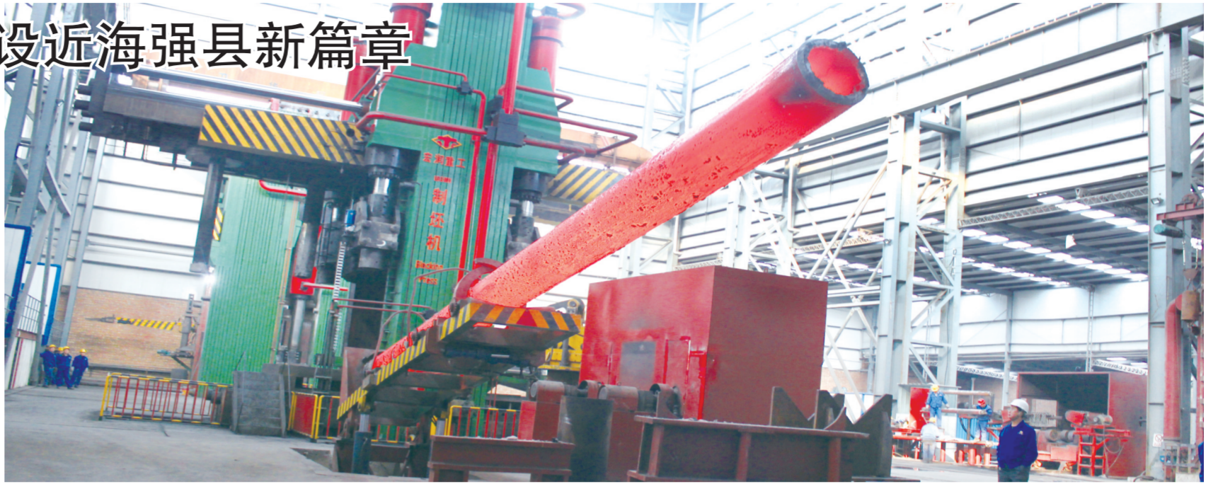
河北宏润核装备科技股份有限公司五万吨设备挤压完成的核电用无缝钢管
